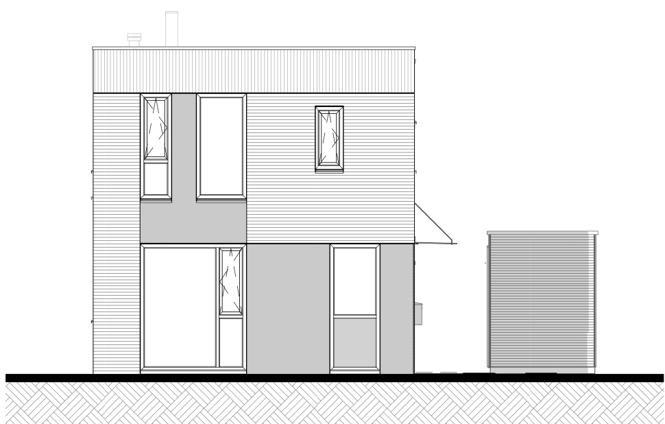
Voorgevel SCHAAL 1 : 100
