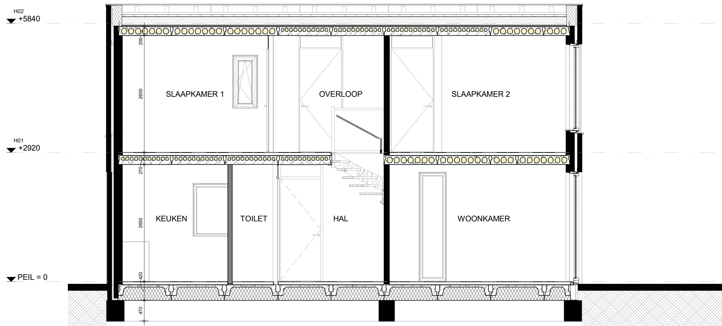
Doorsnede SCHAAL 1 : 50
